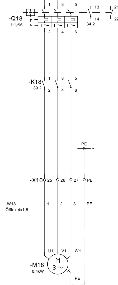
Ausstoßer
